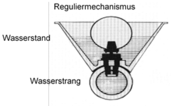
Abb. 1 Querschnitt einer Cuptränke
